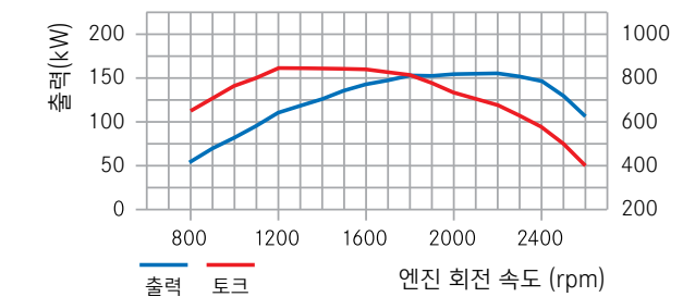
OM934(직렬 4기통) 엔진
