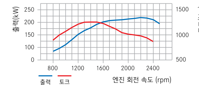
OM936(직렬 6기통) 엔진
