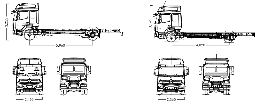
1630L 4X2 빅스페이스
