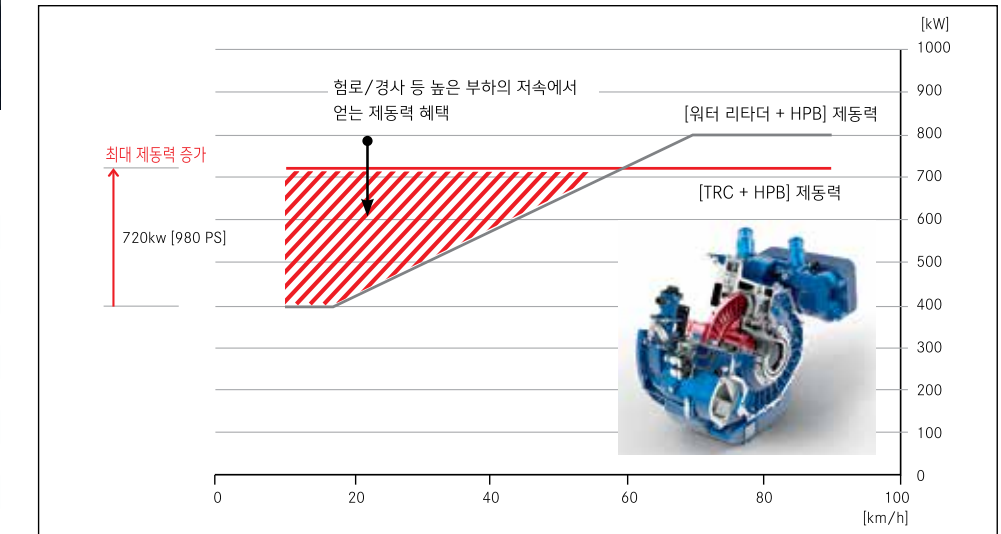
터보 리타더 클러치(TRC) | 초고중량 화물 운송 시에도 수월하게 출발하며, 최대 약 980마력의 정밀하고 획기적인 제동력을 발휘합니다. (3363S 적용)
